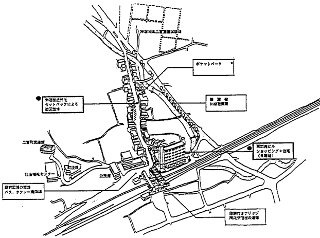
二宮駅北口周辺商店街整備全体構想図
